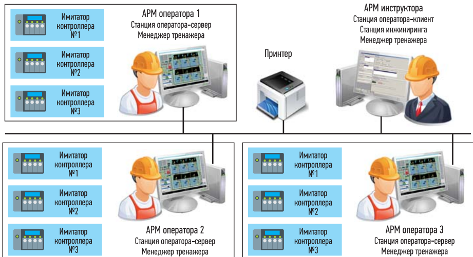
РИС. 2. ▼ Структурная схема КТК для персонала ГРЭС
