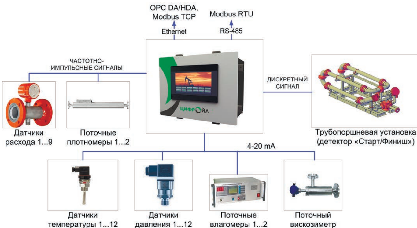
Рис. 2. Схема внешних подключений вычислителя «ЦифрОйл»
