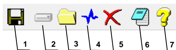
Рисунок 6.2 – Панель инструментов
