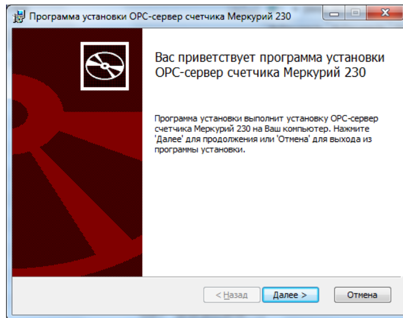
Рисунок 3.1 - Окно инсталлятора
