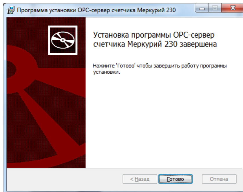
Рисунок 3.6 - Установка завершена
