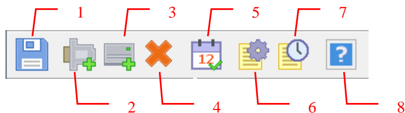
Рисунок 6.2 - Панель инструментов
