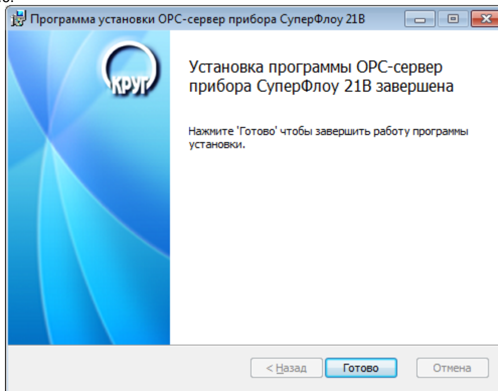
Рисунок 3.6 - Установка завершена
