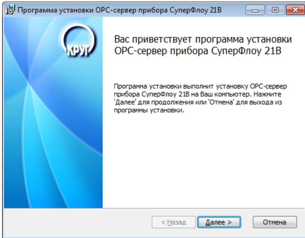
Рисунок 3.1 - Окно инсталлятора
