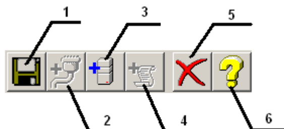
Рисунок 6.2 - Панель инструментов
