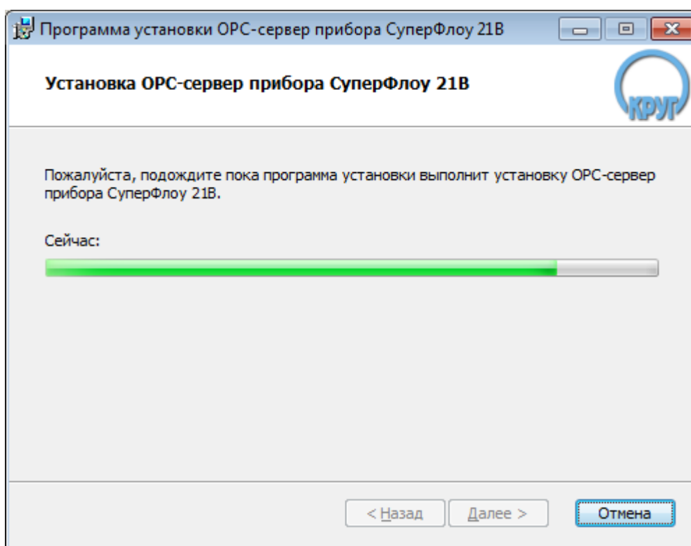
Рисунок 3.5 - Копирование файлов
