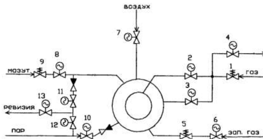
Рисунок 1 - Схема газомазутной горелки
