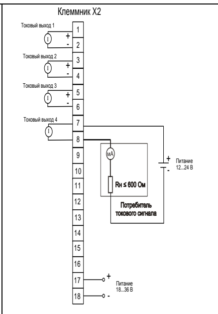
Рисунок 4г – Подключение аналогового выхода, модификация AIO-4/0R
