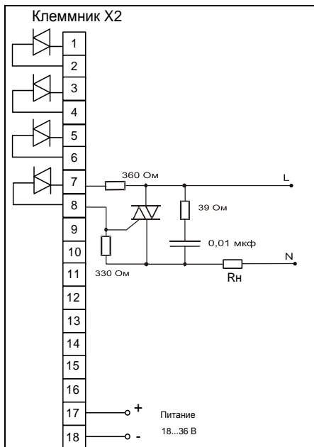
Рисунок 4в – Подключение дискретного выхода, модификация AIO-4/4S
