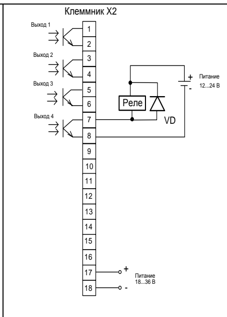
Рисунок 4д – Подключение дискретного выхода, модификация AIO-4/4T
